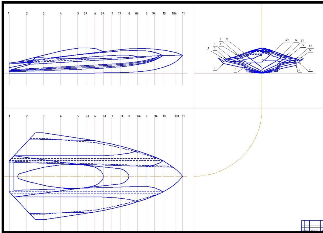
Dronun dizaynı
