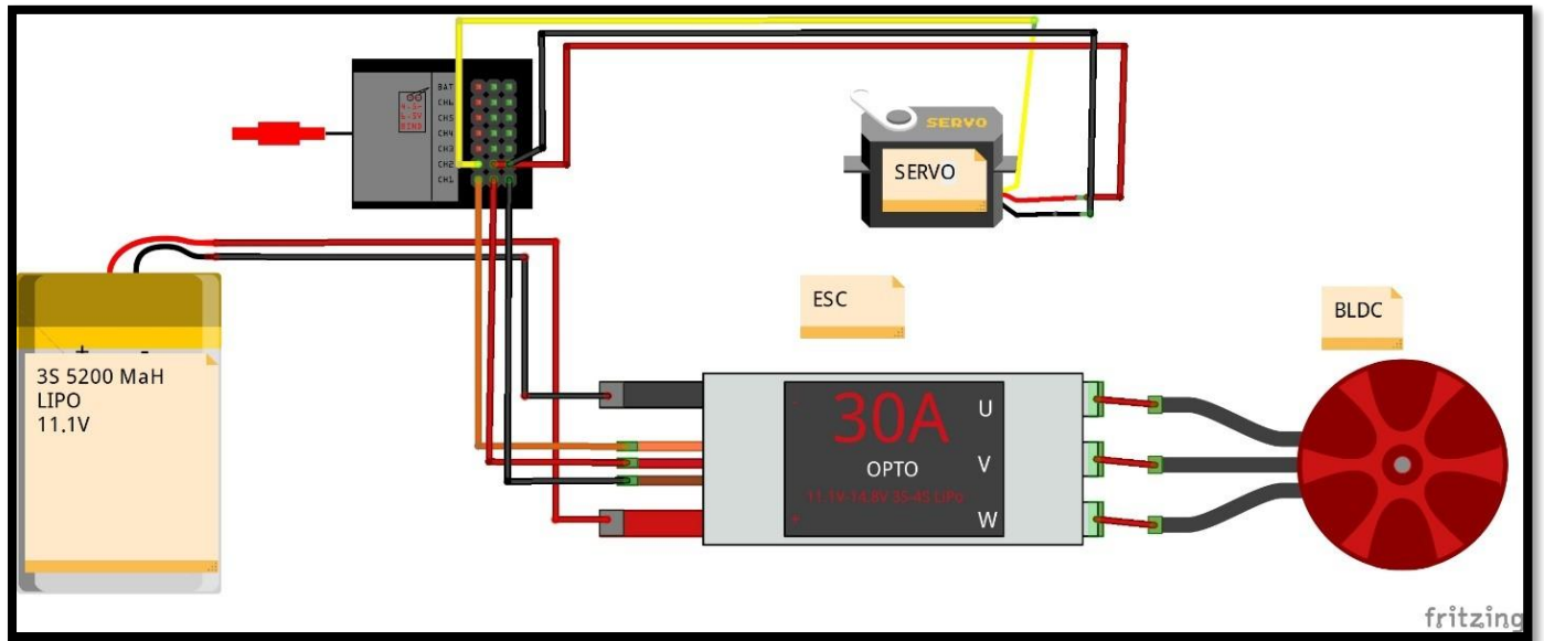
Elektron sxem
