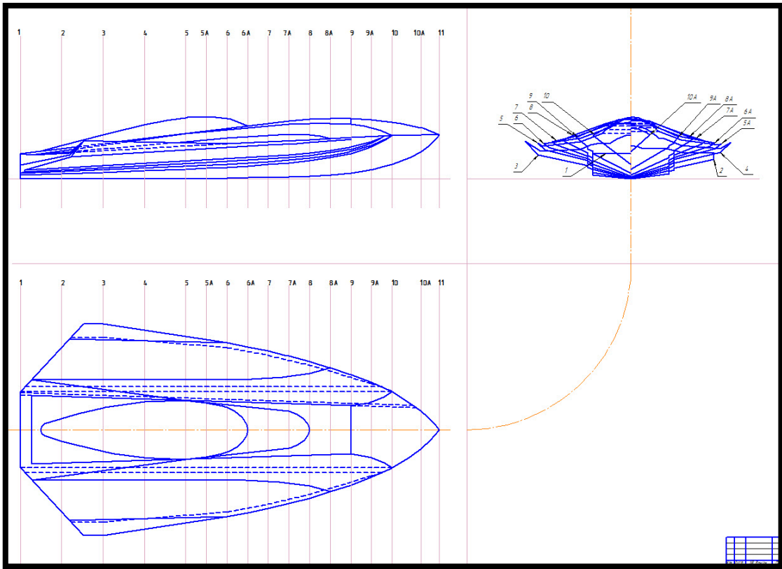
Dronun dizaynı.
